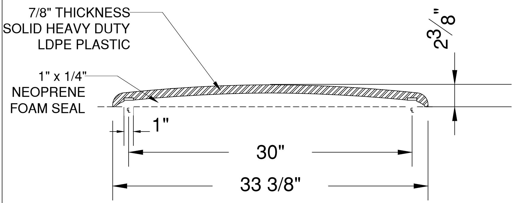
SECTION A-A
